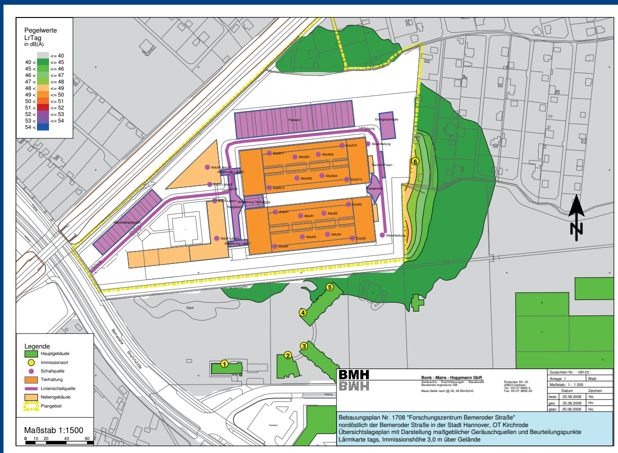
Schallgutachten Tag; Immissionsrichtwert 55 dB(A)
