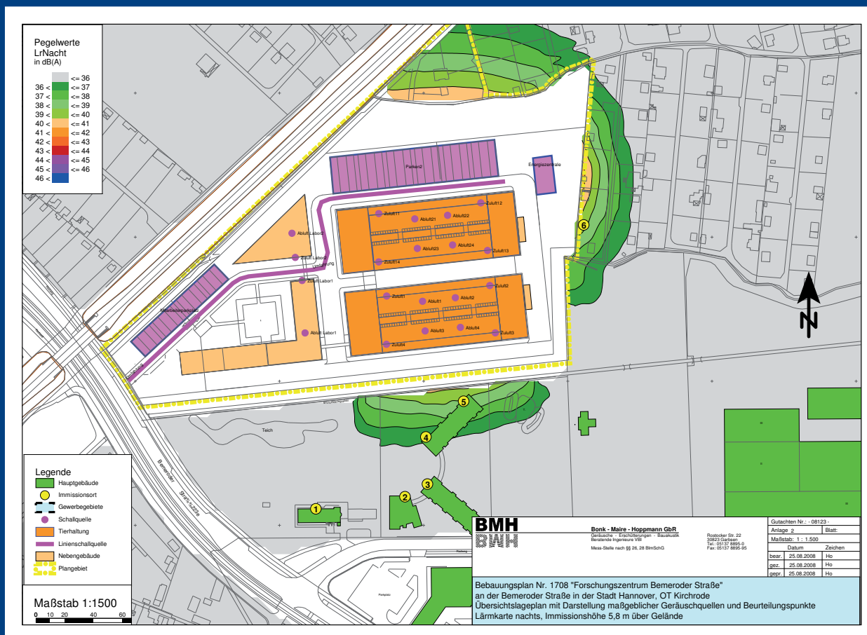
Schallgutachten Nacht; Immissionsrichtwert 44 dB(A)
